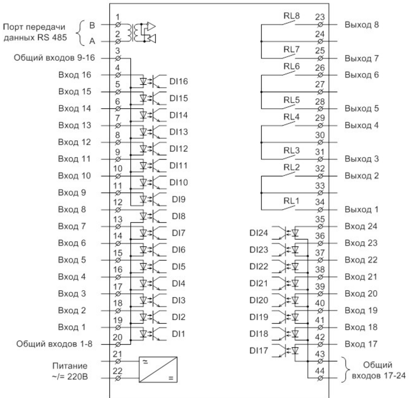
Схема подключения МПУ-ЦС
