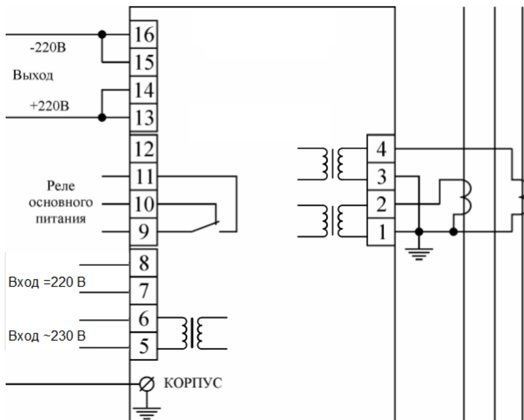
Рисунок Б.1 – Схема подключения Блока
