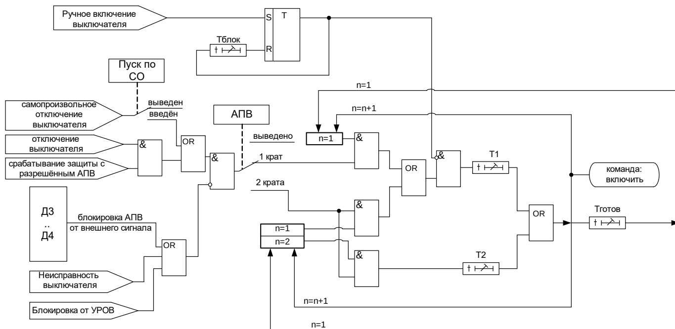
Рисунок 6.7 – Блок АПУ
