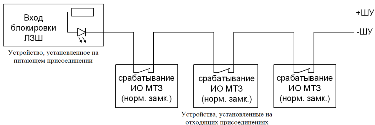
Рисунок 6.12 – Принцип организации логической защиты шин (последовательная схема)
