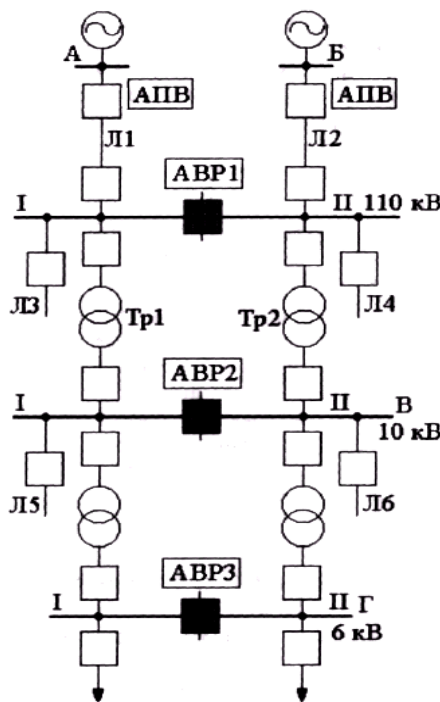
Рисунок 11.10 – Схема нормально разомкнутой распределительной сети с несколькими устройствами АВР и АПВ линий
