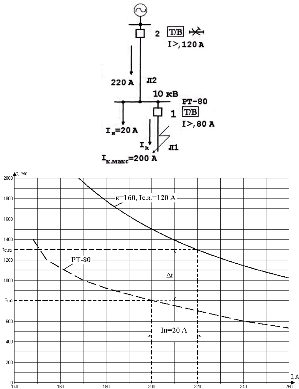
Рисунок 11.6 – Пример согласования характеристик МПЗ-01PRO и дискового индукционного реле РТ-80.
