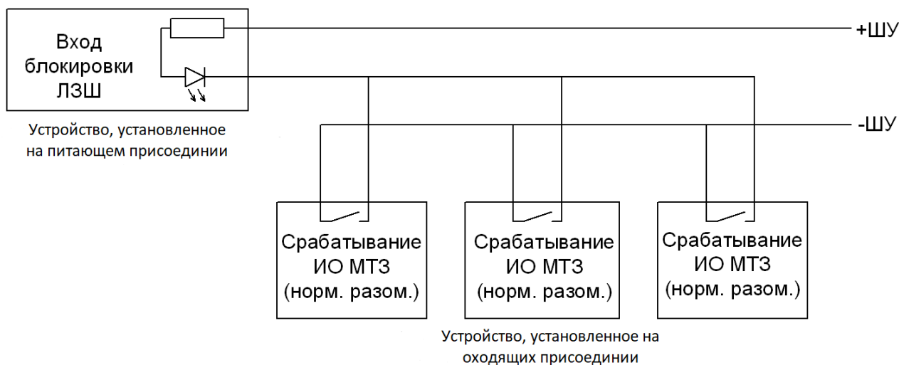
Рисунок 6.11 – Принцип организации логической защиты шин (параллельная схема)
