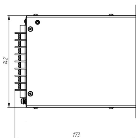
Габаритные и присоединительные размеры
