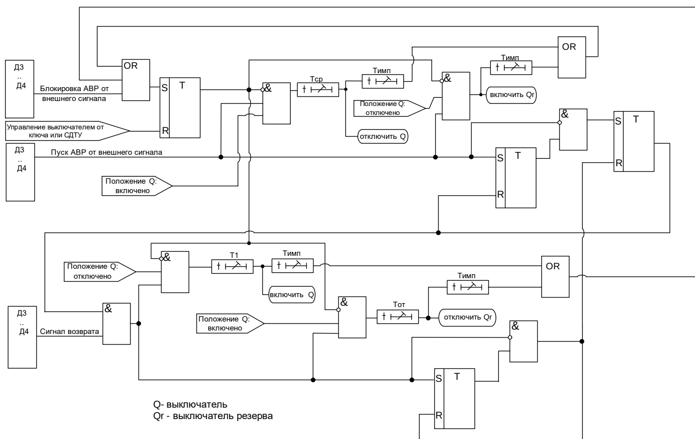
Рисунок 6.10 – Блок АВР
