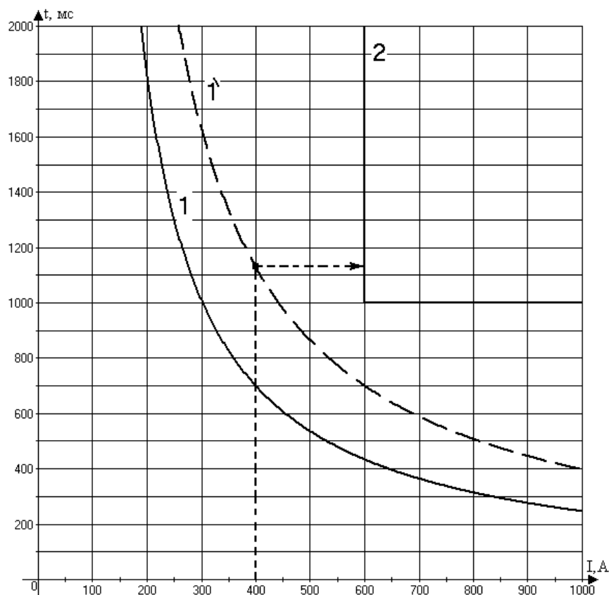
Рисунок 11.8 – Пример согласования обратнозависимой характеристики МПЗ-01PRO и не-зависимой характеристики МТЗ последующего элемента
