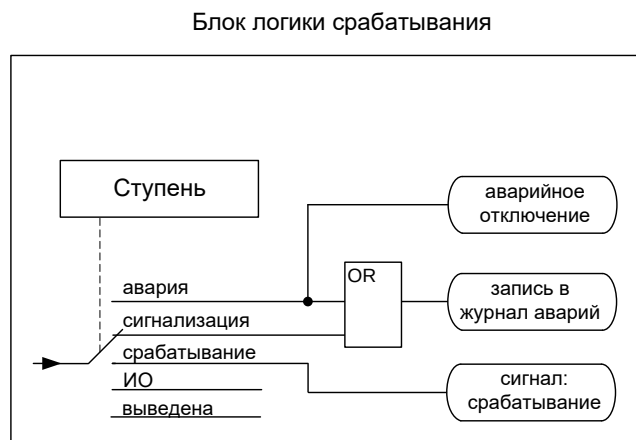
Рисунок 6.3 – Блок МТЗ при междуфазных КЗ (блок входной логики, таймер и блок логики срабатывания)
