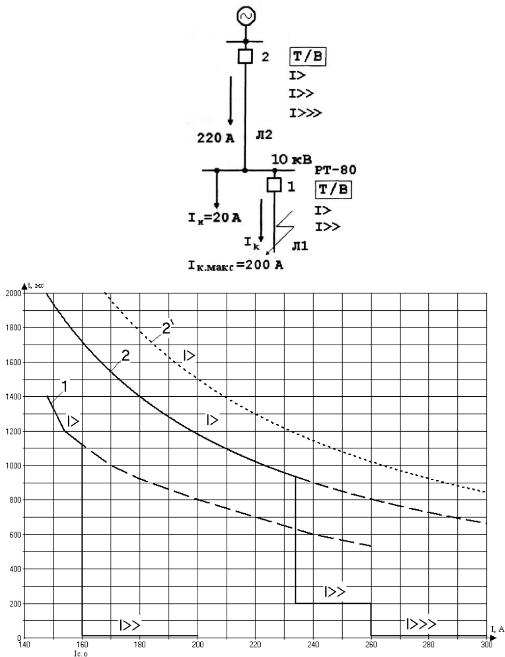
Рисунок 11.7 – Пример согласования характеристик МПЗ-01PRO и реле РТ-80 с использованием "отсечки".
